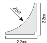
寸法図
